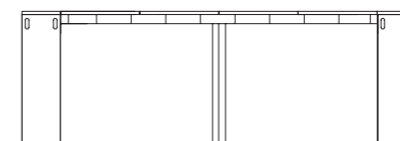
Apertura massima / Max extension cm 225 (45 + 4 x 45) x 90 x h 75
