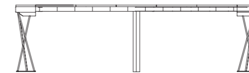
Apertura massima / Max extension cm 270 (45 + 5 x 45) x 120 x h 75
