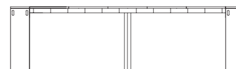
Apertura massima / Max extension cm 270 (45 + 5 x 45) x 90 x h 75
