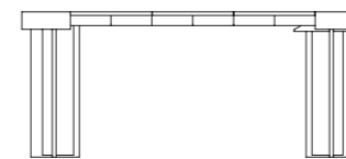
Aperto (3 allunghe) / Open (3 extensions) 110 × 176 × h 75 cm
